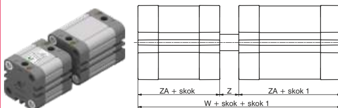
Tandem przeciwstawny ze wspólnym tłoczyskiem
