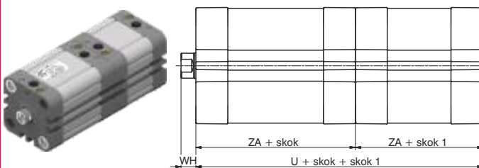
Tandem pchający z niezależnymi tłoczkami
