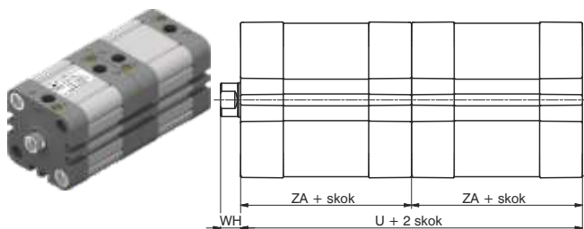
Tandem pchający ze wspólnym tłoczyskiem
