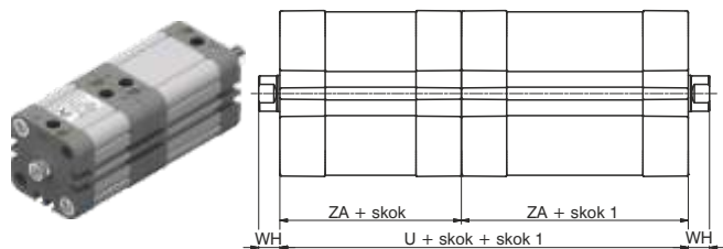
Tandem z przeciwstawnymi tłoczkami
